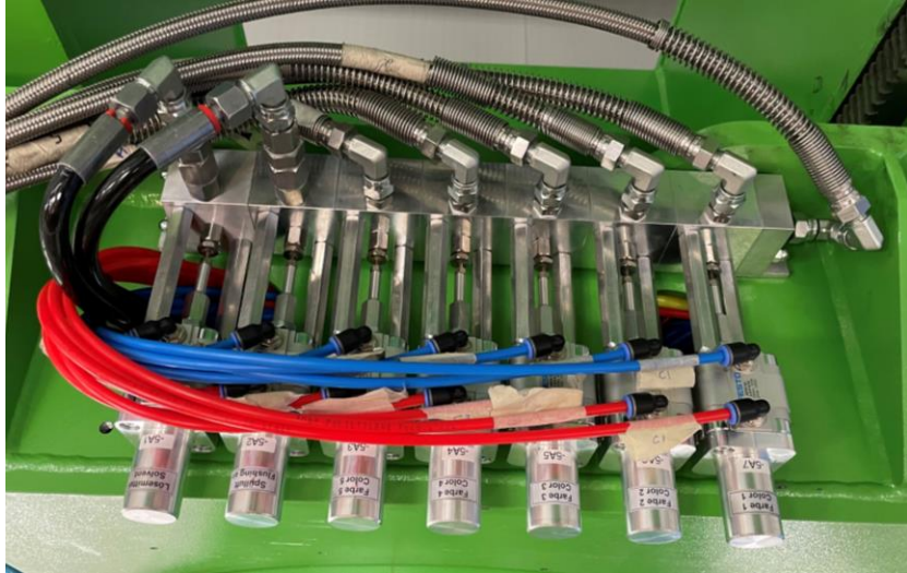
Bild zeigt einen 5-fach Farbwechselblock Picture shows a 5-colour change block
